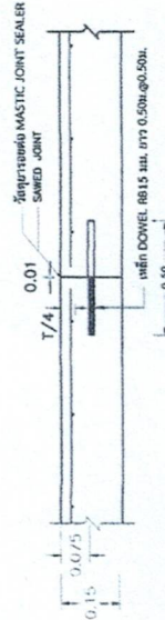
CONTRACTION JOINT ขนาดตามจริง (NOT SCALE)
